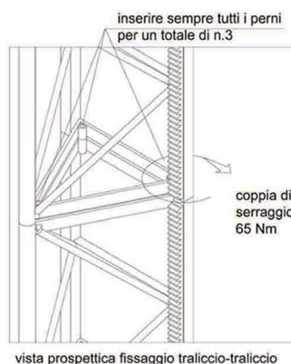
vista prospettiva fissaggio traliccio-traliccio
